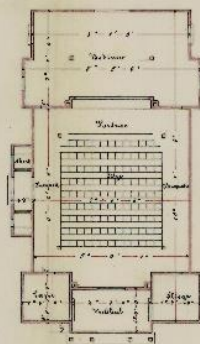
AUFRISS
